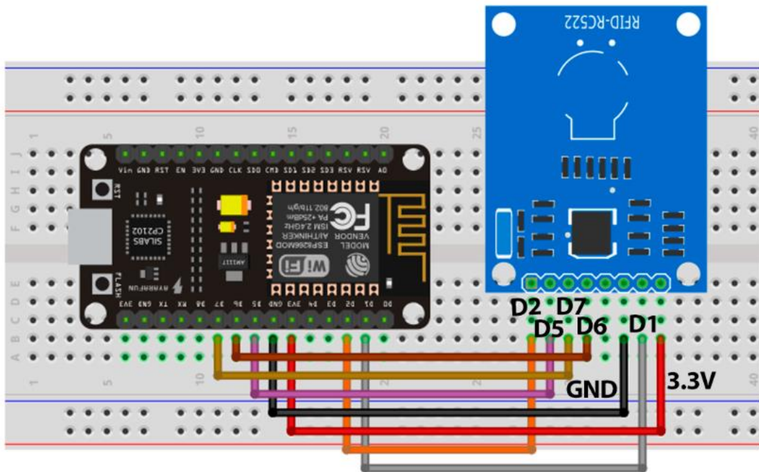
Diagrama do Módulo RFID MFRC522 com NodeMCU
